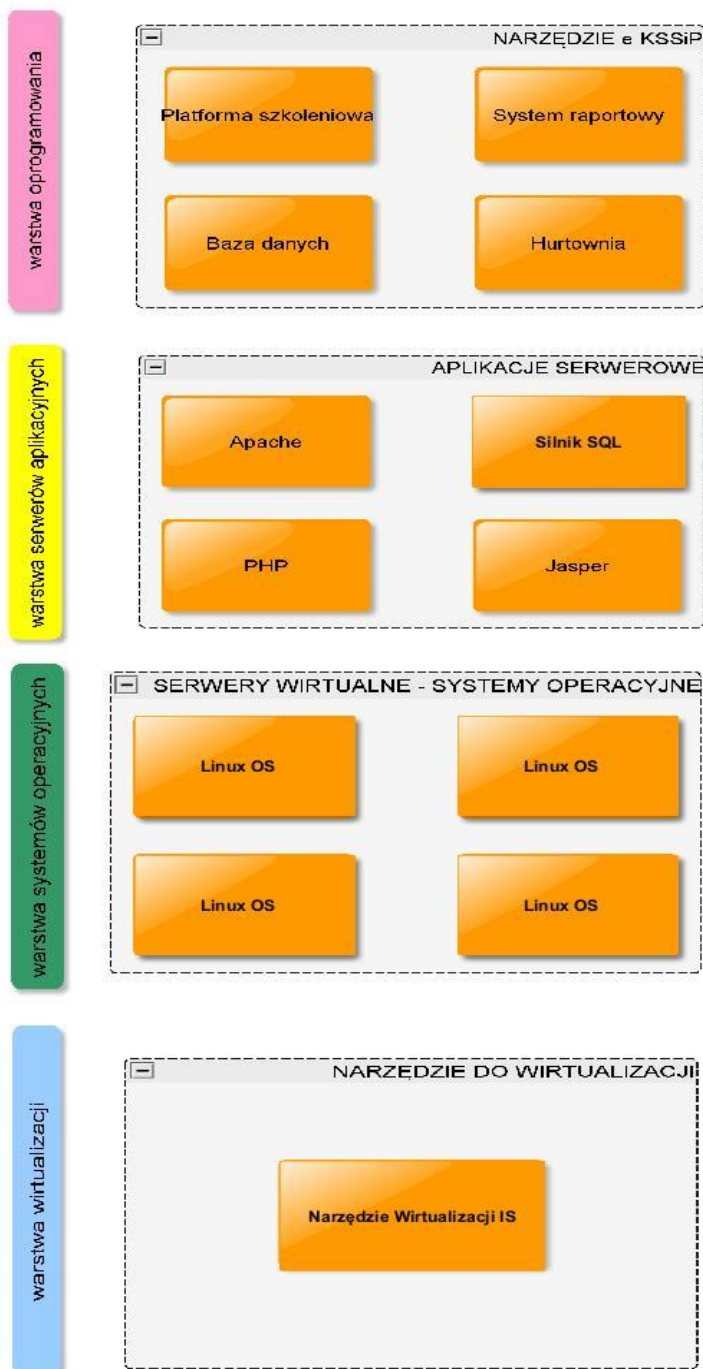
Rysunek 3. Warstwy logiczne Platformy Szkoleniowej e-KSiP.
