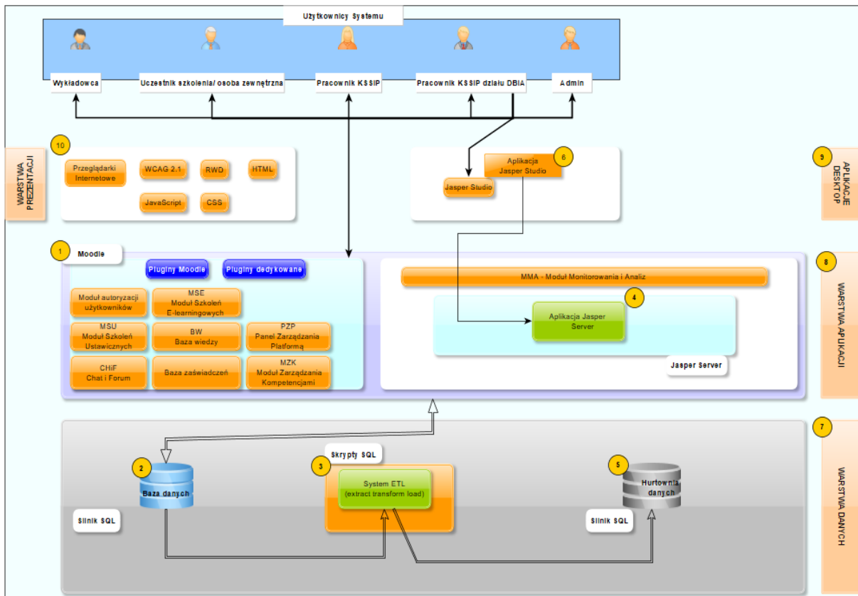
Rysunek 1. Architektura Platformy Szkoleniowej e-KSSiP
