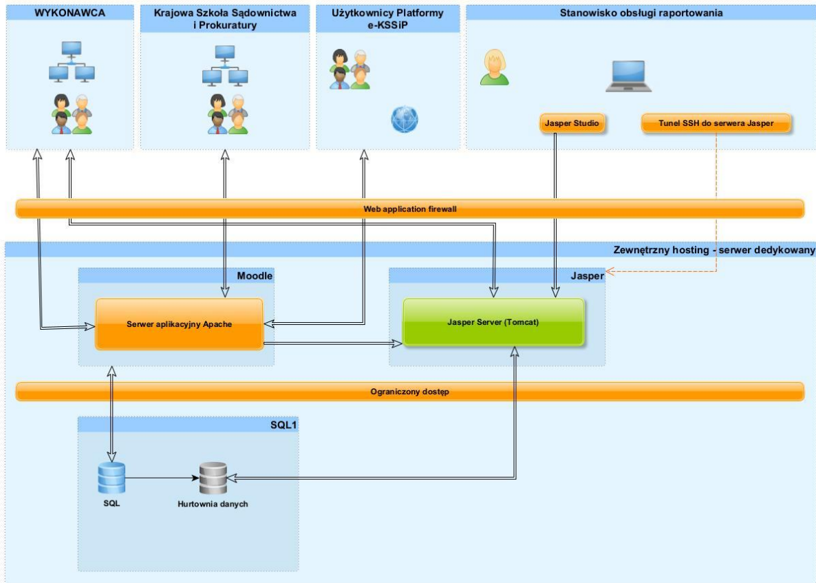
Rysunek 2. Przepływ danych
